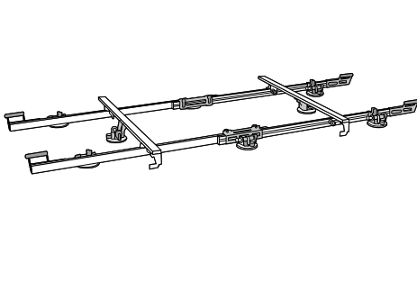
Handling frame equipped with suction cups Telaio di movimentazione dotato di ventose Châssis doté de ventouses Transportrahmen mit Saugnäpfen
